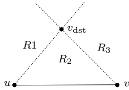
FIG. 2.5. The proof of Lemma 2.3.
