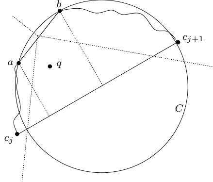
FIG. 3.5. The proof of Lemma 3.4.
